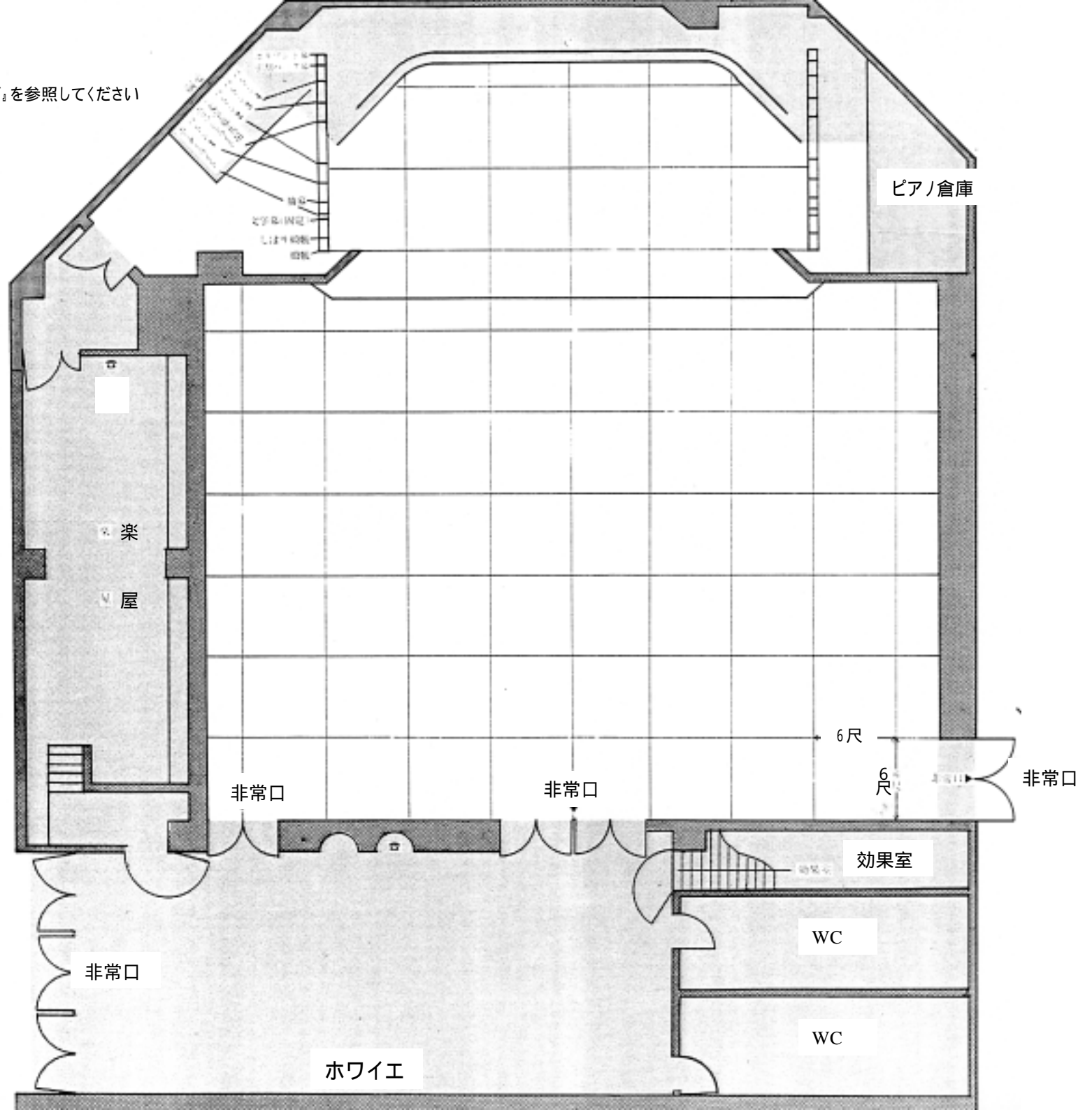
花巻市文化会館中ホール平面図 1/100
